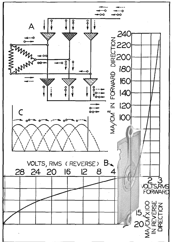
Fig. 2—High-Voltage Selenium Rectifier Plate.
