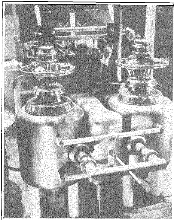
Fig. 15—Final Amplifier.
