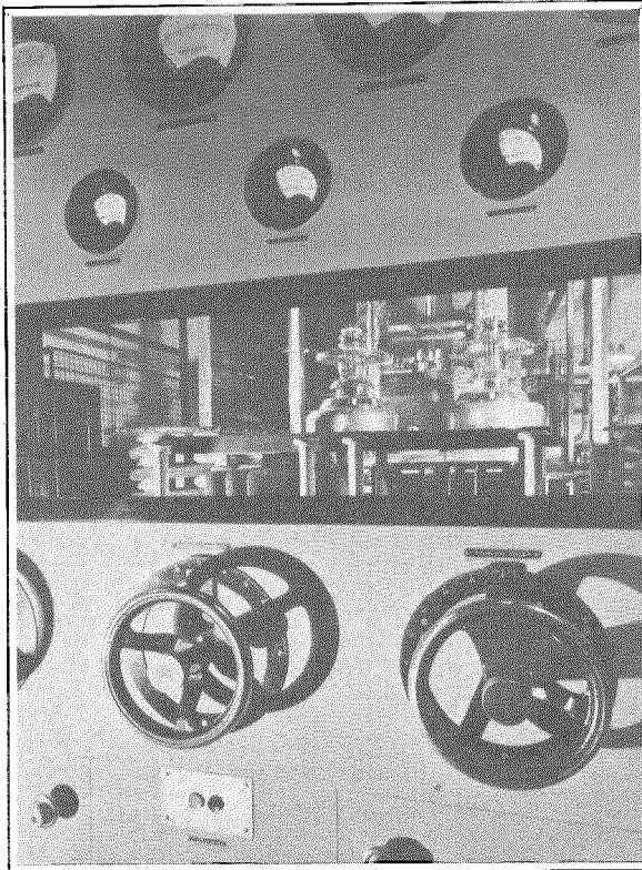
Fig. 16—Front Panel—Final Amplifier.
