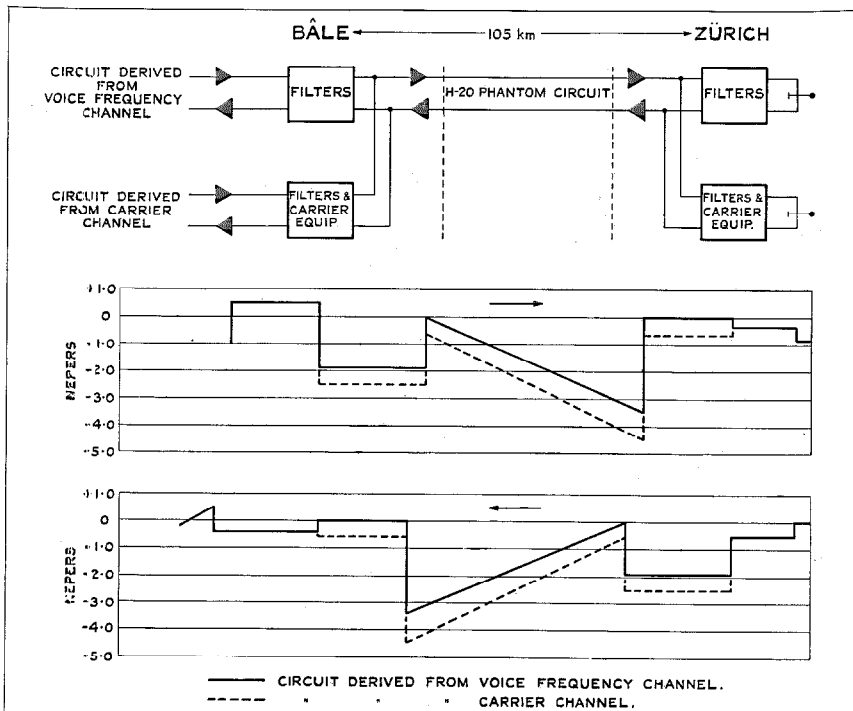
Fig. 12—Level Diagram.
