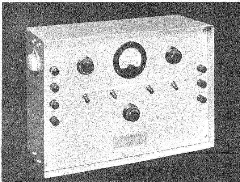
Fig. 1—Amplifier.
