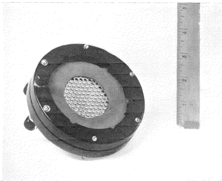
Fig. 6—Coupler.
