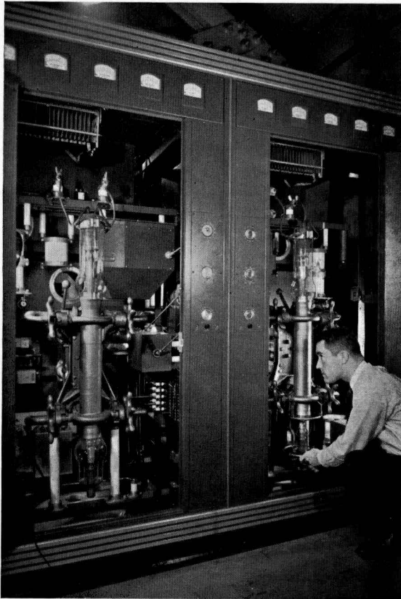
Fig. 5—50-kW Amplifier.
