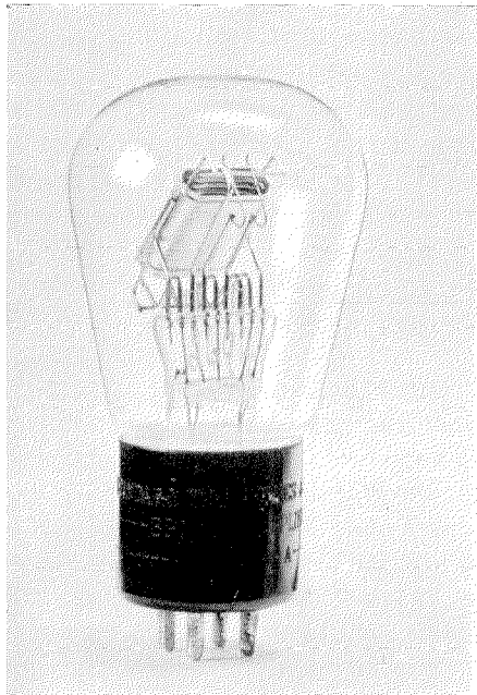
Figure 1-a—No. 4019-A Type Tube
