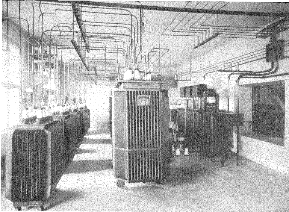
Figure 13—20,000 Volt Rectifier.
