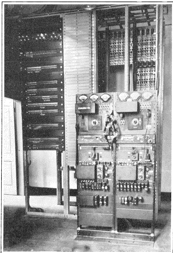
Repeaters—Chillán.
