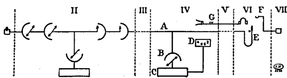
Fig. 18—Diagramme d'établissement d'une communication automatique vers manuel. Indicateur d'appels tandem sans monocorde
