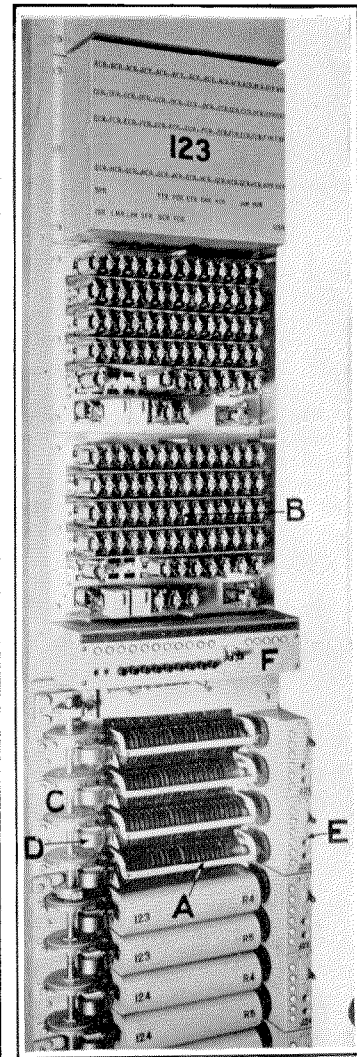
Fig. 14—Détails Fig. 13 et 14.—Vues d'ensemble et détails d'une baie d'enregistreur à relais (type Nantes)
