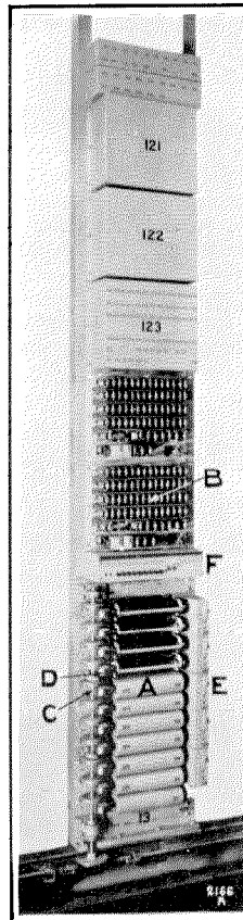
Fig. 14—Détails Fig. 13 et 14.—Vues d'ensemble et détails d'une baie d'enregistreur à relais (type Nantes)
