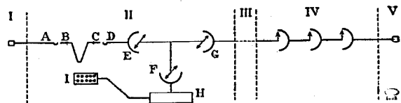
Fig. 19—Diagramme d'établissement d'une communication manuel vers automatique. Sélection directe I, Abonné demandeur;—II, Bureau manuel de départ;—III, Ligne auxiliaire;—IV, Bureau automatique d'arrivée;—V, Abonné demandé.
