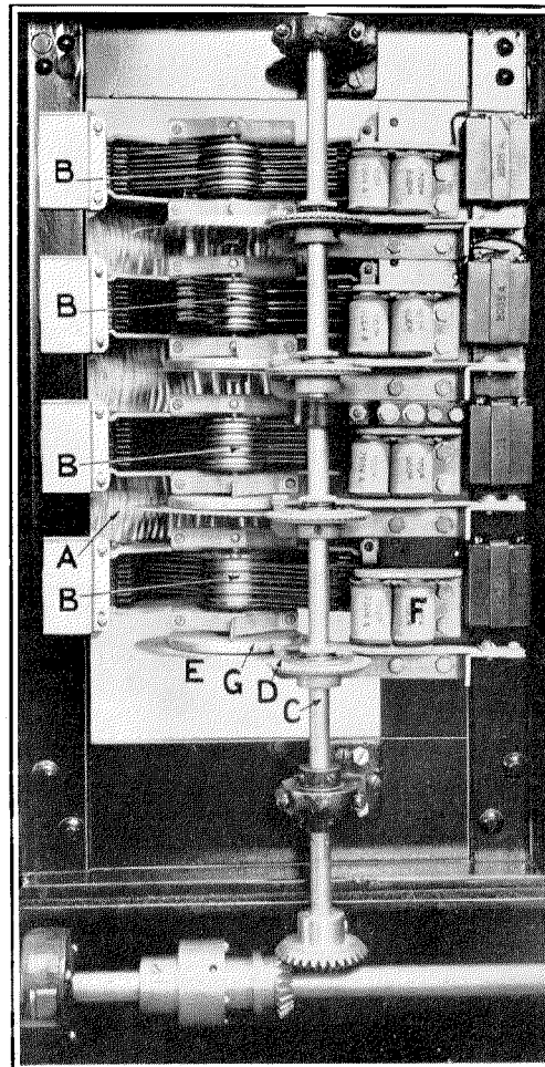
Fig. 4—Vue avant d'une baie de chercheurs A, Multipliage en câbles-rubans;—B, Chariots porte-balais;—C, Arbre en rotation permanente;—D, Roue motrice;—E, Roue entraînée flexible;—F, Electro d'embrayage;—G, Tambour numéroté.
