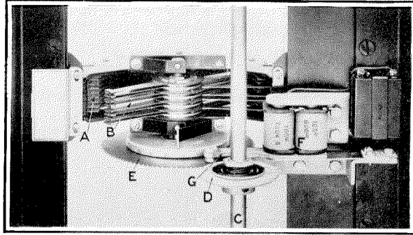
Fig. 3—Vue d'un chercheur A, Banc de contacts;—B, Balais;—C, Arbre en rotation permanente;—D, Roue motrice;—E, Roue entraînée flexible;—F, Electro d'embrayage;—G, Armature de l'électro d'embrayage.
