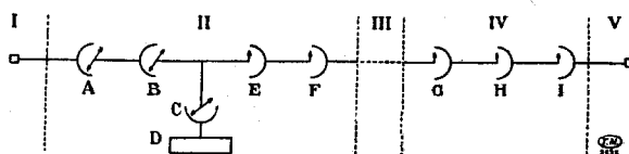
Fig. 2—Diagramme d'établissement d'une communication entre deux abonnés reliés à des bureaux automatiques différents
